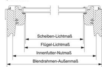
Längsschnitt
