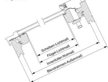
Längsschnitt
